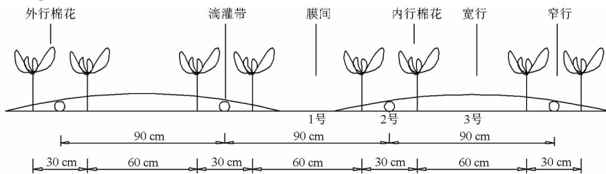
图 1 一膜两带四行种植模式与土壤取样点示意图
